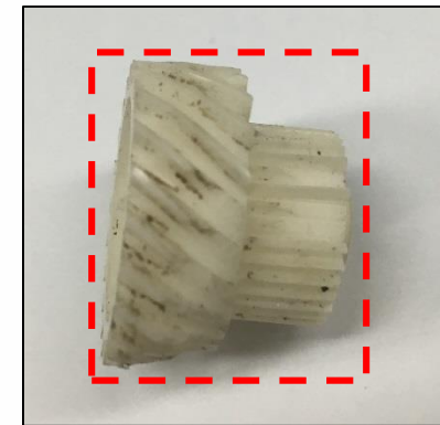
<파손 기어>
