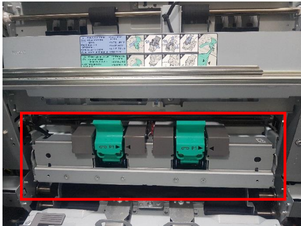
3 Stapler assembly 제거(나사2개, 커넥터1개)
