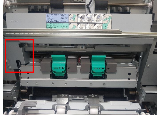
2. 고정 철판 제거(나사 2개, LEFT VIEW)
